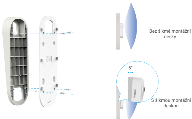
Obr. 2 Šikmá montážní deska 2
