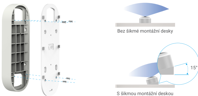
Obr. 1 Šikmá montážní deska 1
