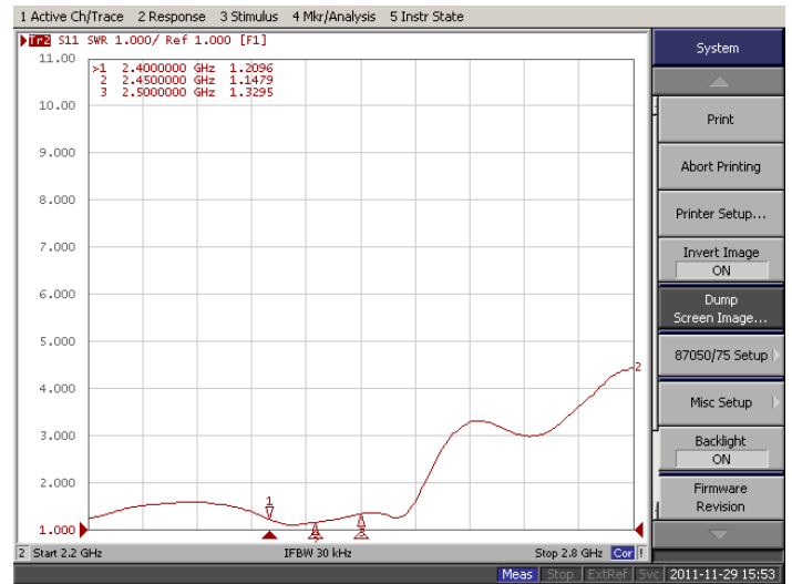
V.S.W.R
